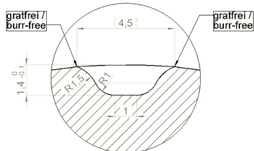
DETAIL C 10 : 1
